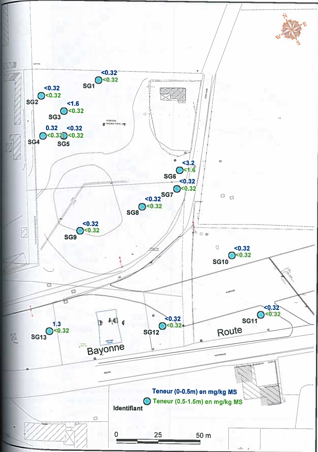
Figure 4 : Répartition des teneurs en hydrocarbures aromatiques polycycliques (somme des 16 EPA)
